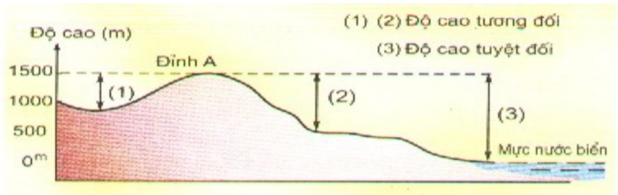
Hình 34. Độ cao tuyệt đối và độ cao tương đối
