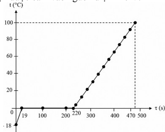
Hình I.2. Đồ thị nhiệt độ - thời gian
