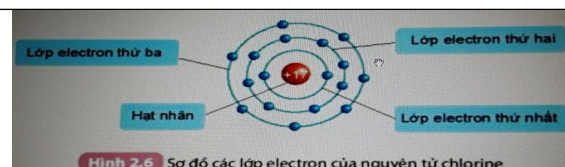
Hình 2.6 Sơ đồ các lớp electron của nguyên tử chlorine
