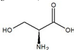
L - serine
