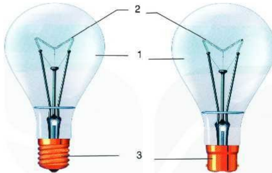
Cấu tạo của bóng đèn sợi đốt
