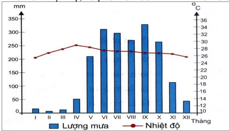
BIỂU ĐỒ NHIỆT ĐỘ, LƯỢNG MƯA CỦA THÀNH PHỐ HỒ CHÍ MINH
