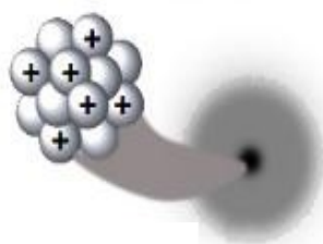
Nguyên tử carbon
