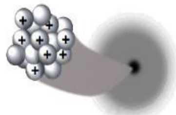
Nguyên tử oxygen
