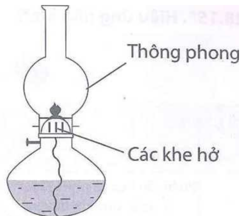
Hình 28.1. Đèn dầu
