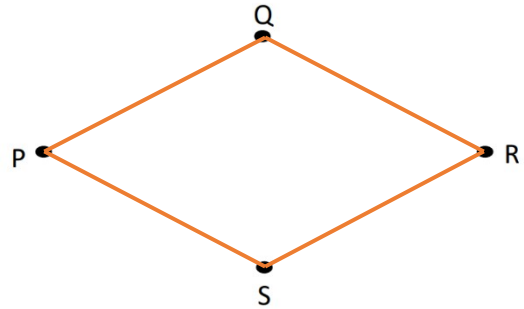
Hình thoi PQRS
