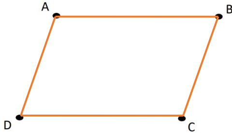
Hình bình hành ABCD
