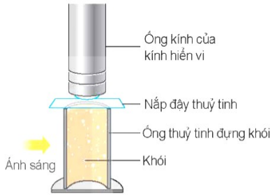
Hình 8.1. Sơ đồ thí nghiệm quan sát chuyển động Brown trong không khí
